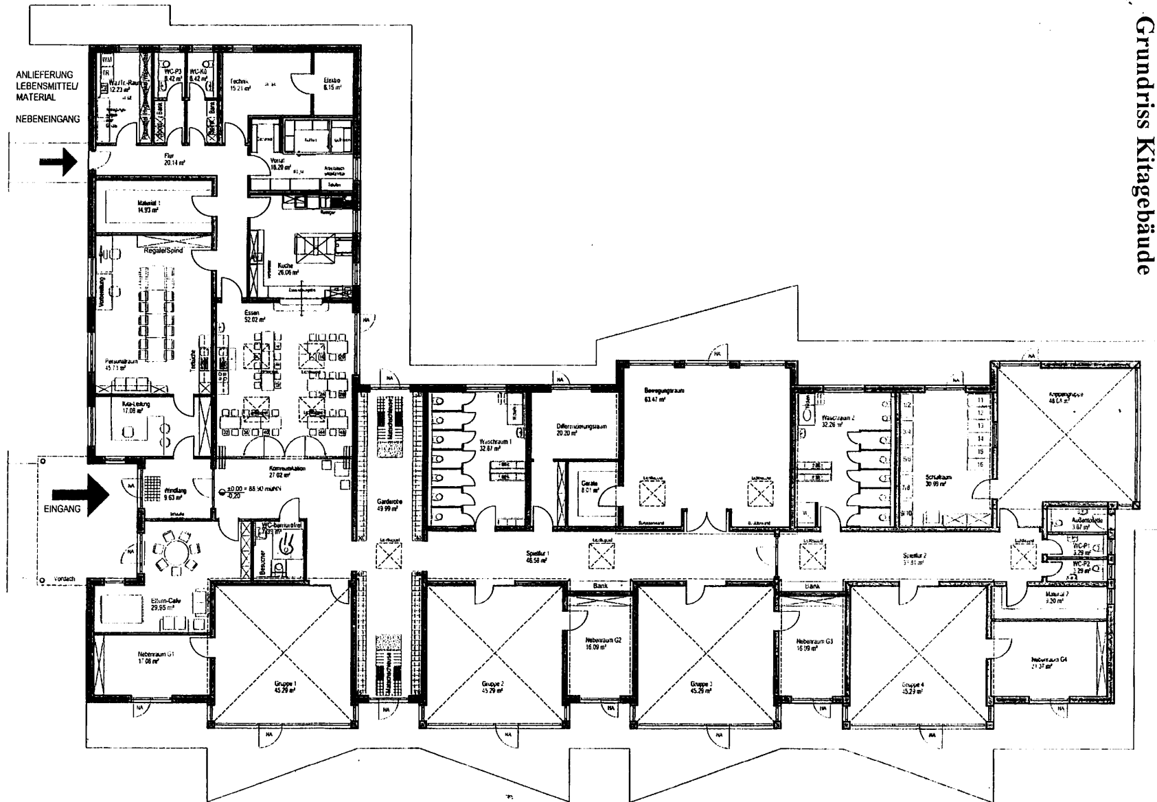
GRUNDRISS ERDGESCHOSS, Architekturbüro Walter Schweitzer
