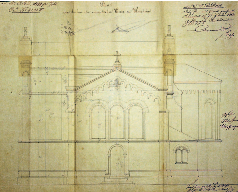
Kirchenbauplan 1861 (Südseite)
