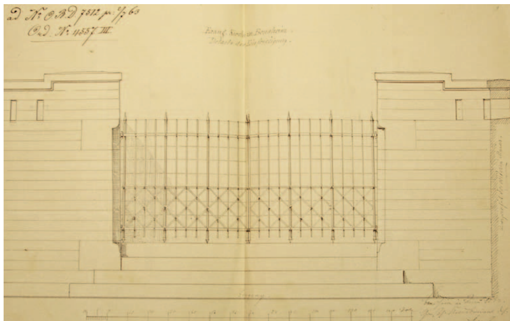
Kirchenbauplan 1863 (Details der Einfriedigung)
