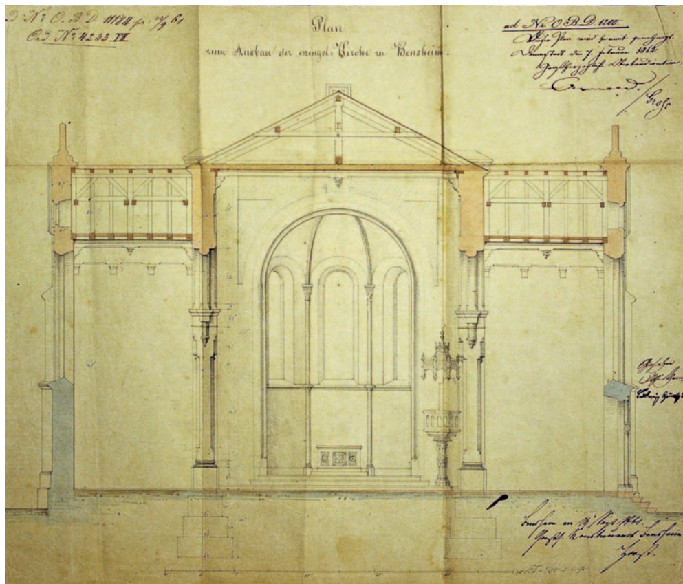
Plan 1861 Innenansicht Chorraum
