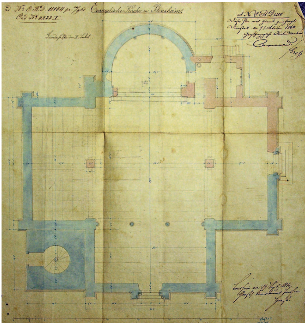
Grundriss von 1861
