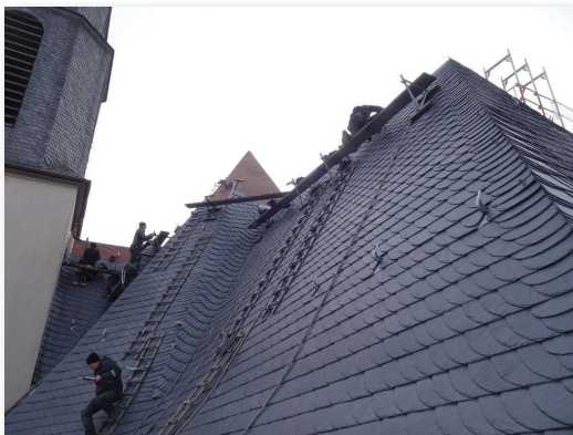
Stand der Schieferarbeiten auf der Nordwestseite mit Empore, Feb. 2026
