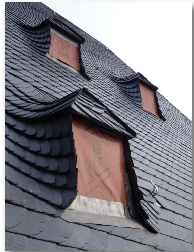
Eingebaute Dachgauben auf der südlichen Hauptdachfläche
